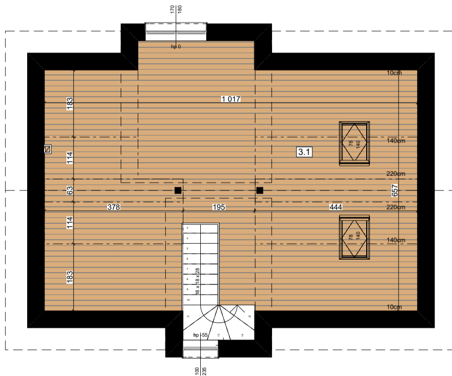
RZUT PODDASZA
